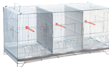
90cm Cod. 90669 ✦ cm: 90 x 34 x 43 h 🐦 4 Ud.
