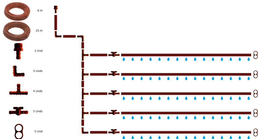
Kit de irrigación - Huerto Irrigation kit - Vegetable garden Cod. 90882
