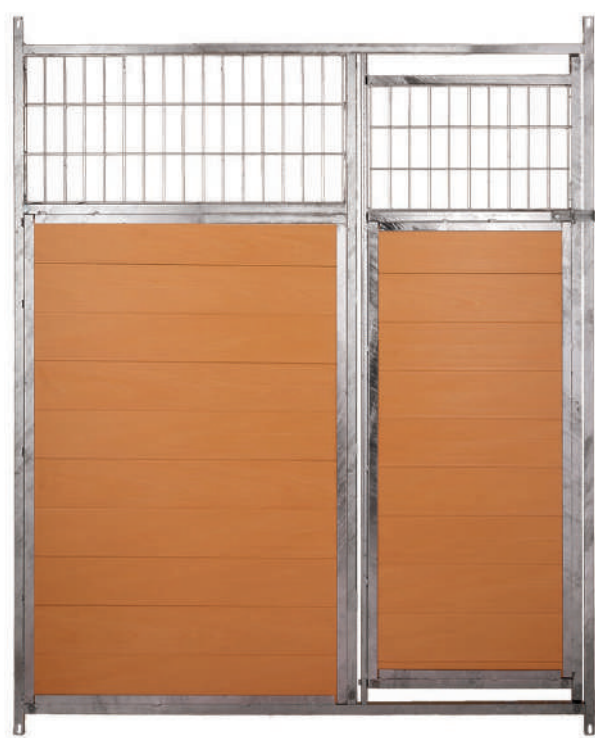
Mixto con puerta Cod. 70973 cm.: 150 x 185 h.
