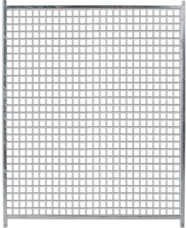
Malla 5x5 cm. Cod. 70294 cm.: 100 x 184 h. Cod. 70295 cm.: 150 x 184 h. Cod. 70296 cm.: 200 x 184 h.
