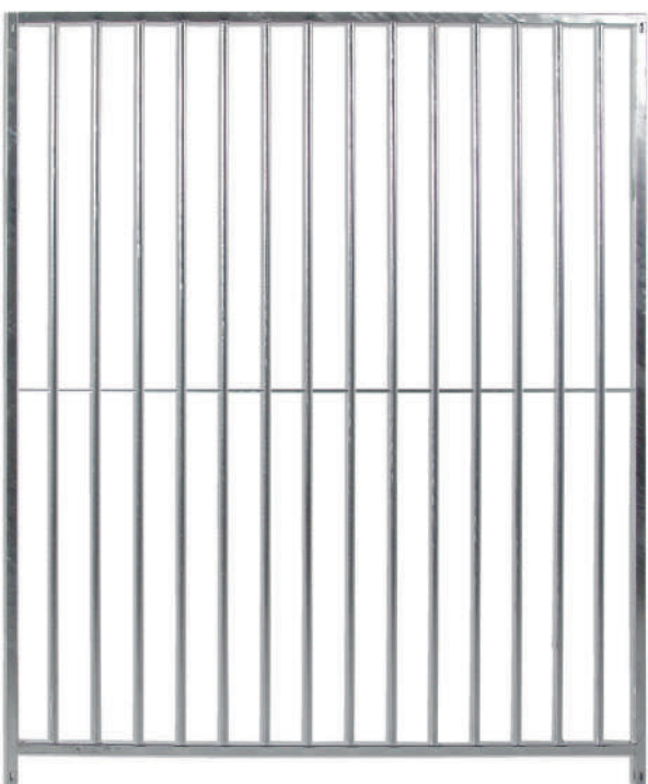
Barras Cod. 70286 cm.: 100 x 184 h. Cod. 70287 cm.: 150 x 184 h. Cod. 70288 cm.: 200 x 184 h.
