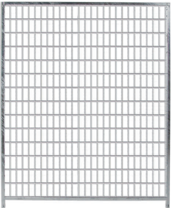
Malla 5x10 cm. Cod. 70298 cm.: 100 x 184 h. Cod. 70299 cm.: 150 x 184 h. Cod. 70300 cm.: 200 x 184 h.
