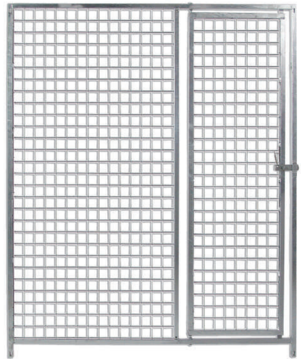
Malla 5x5 cm. con puerta Cod. 70278 cm.: 100 x 184 h. Cod. 70279 cm.: 150 x 184 h. Cod. 70280 cm.: 200 x 184 h.
