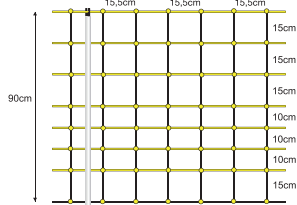
Malla eléctrica ovino 0,90 x 50m Electric mesh for sheep 0,90x50m
